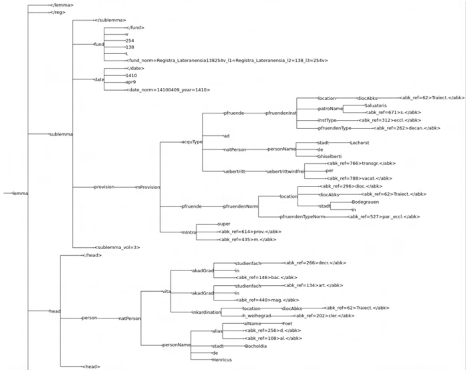
Abb. 2: Parse tree : Regest aus dem RG Online („Henricus de Bocholdia“; RG III, Sp. 14, 9. April 1410) und semantische Erschließung via ANTLR.
