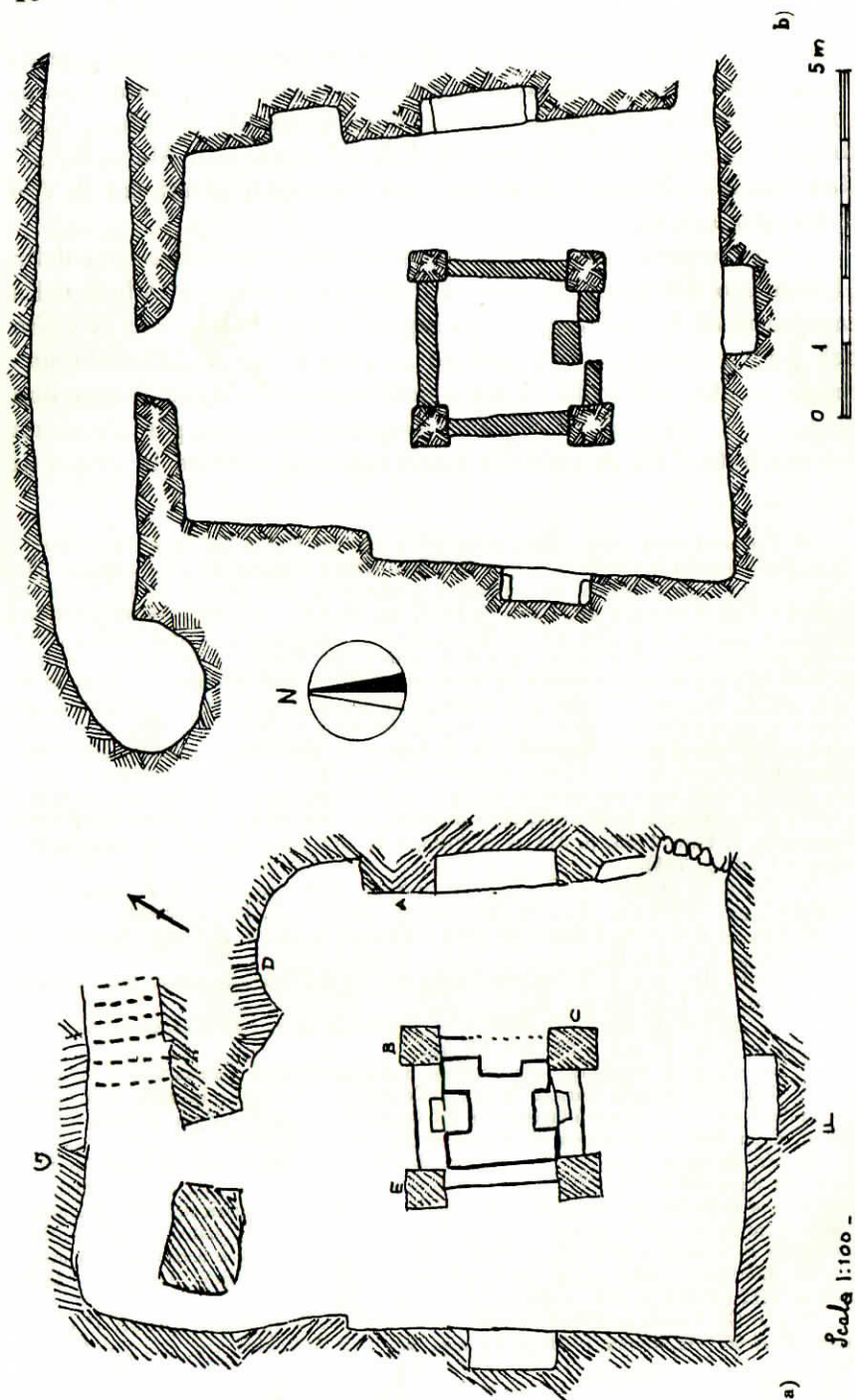
FIG. 2. — Planimetria della cripta della Madonna o dei Santi in località Petracca (Noto), secondo P. Orsi (a) e secondo G. Sluga (b).
