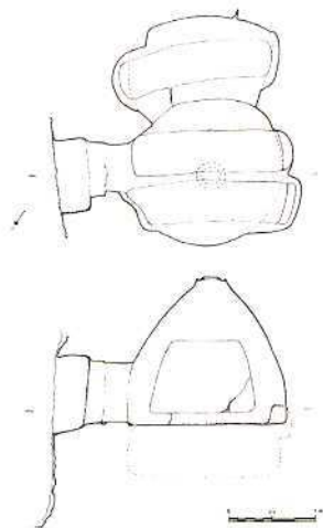
Tav. XII . Scalepiane. Tomba a tholos
