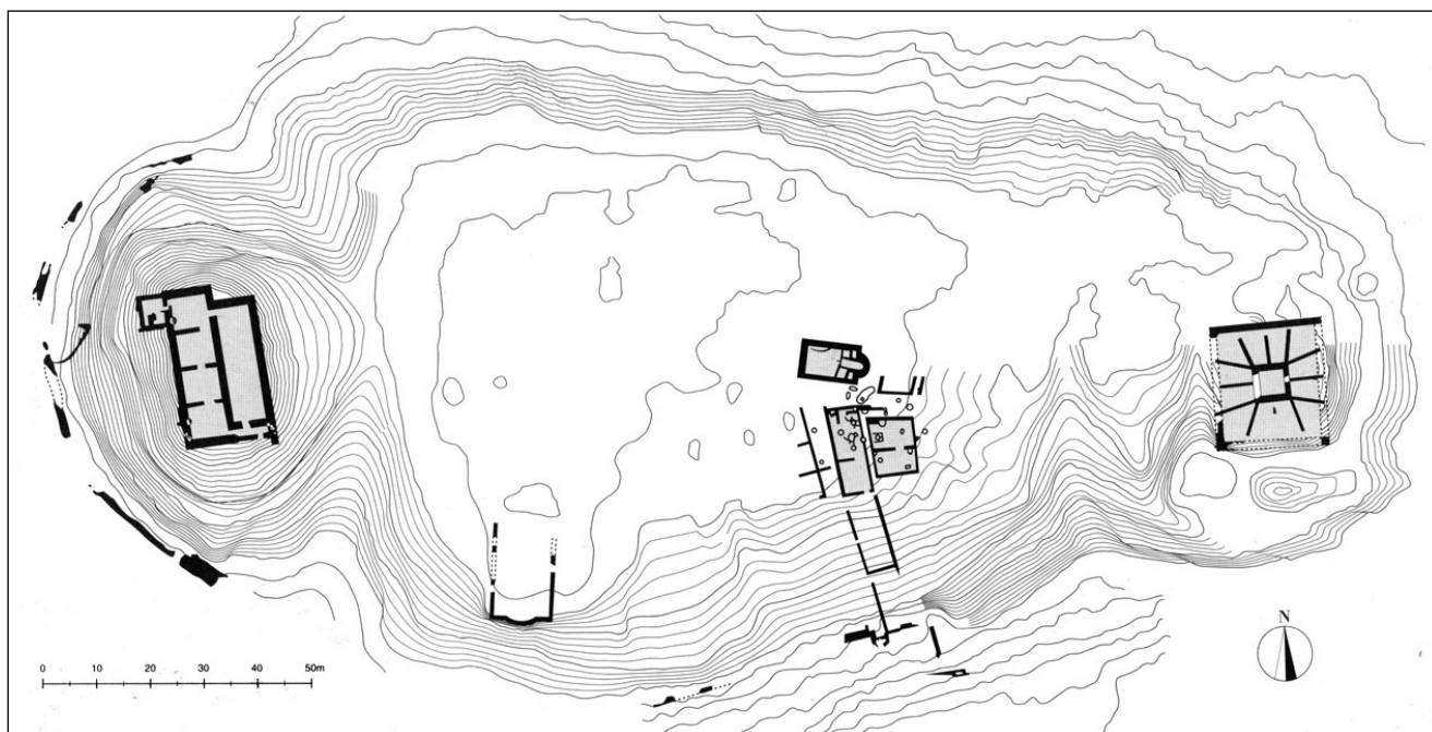
fig. 3a – Fiorentino. Planimetria generale del sito: sulla sinistra il palatium , al centro in basso la cattedrale, sulla destra la torre (da PIPONNIER 2000).
